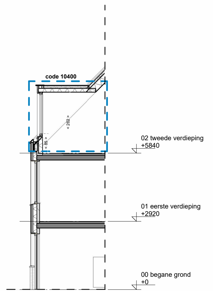
doorsnede
