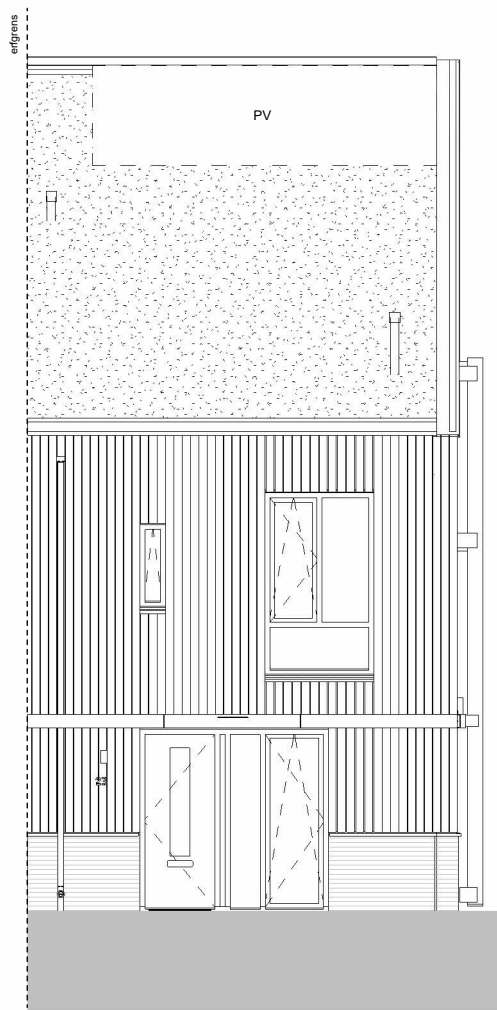
voorgevel
