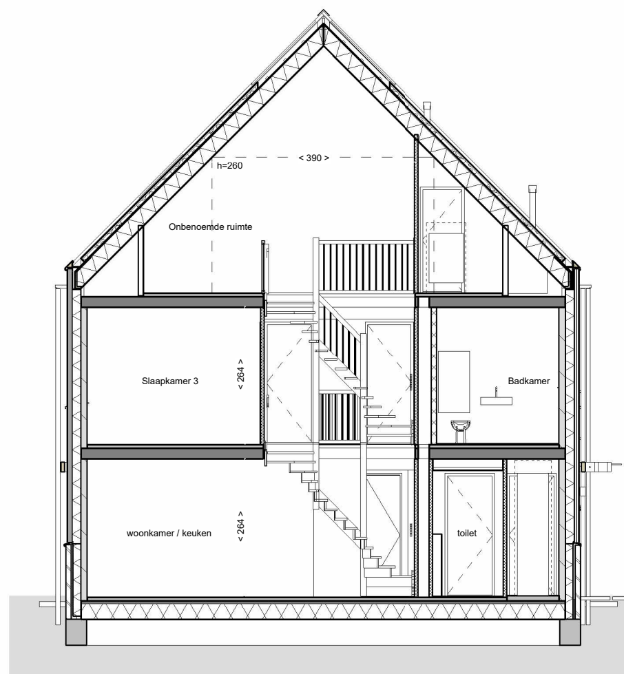
doorsnede
