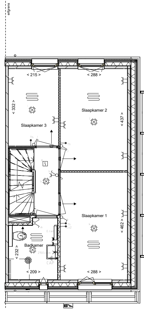
01 eerste verdieping
