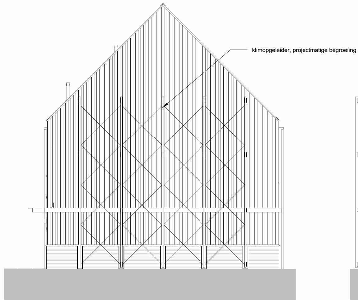
kopgevel
