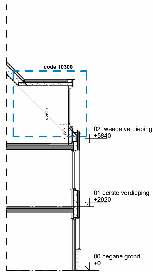
doorsnede
